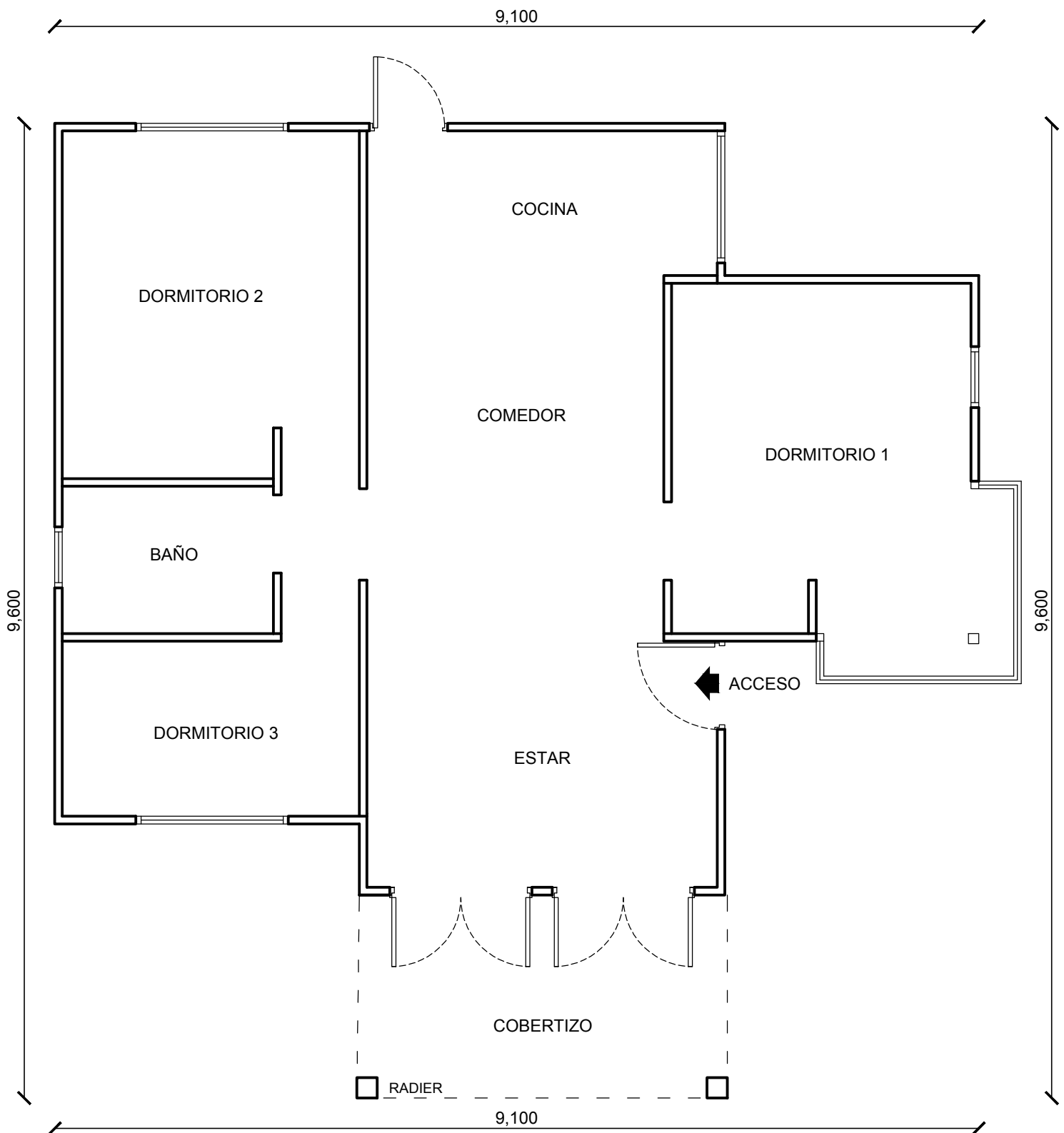
PLANO DE DISTRIBUCIÓN CASA MODELO JUAN PABLO 61m 2
